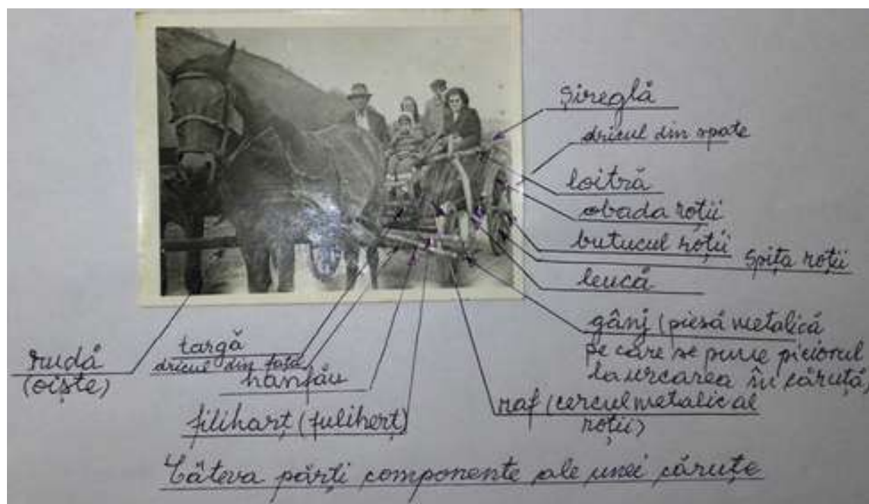
F . 35 .Căruță – părți componente
