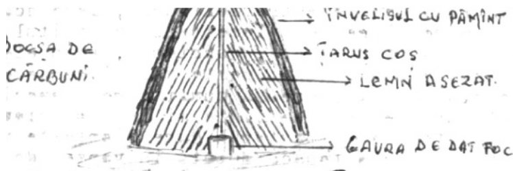
Schiță bocșă de cărbuni (Nicolae Lădar, Manuscris )
