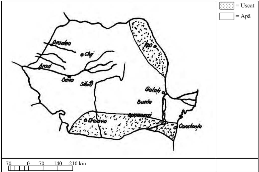
Foto 1. Situația în Precambrian
