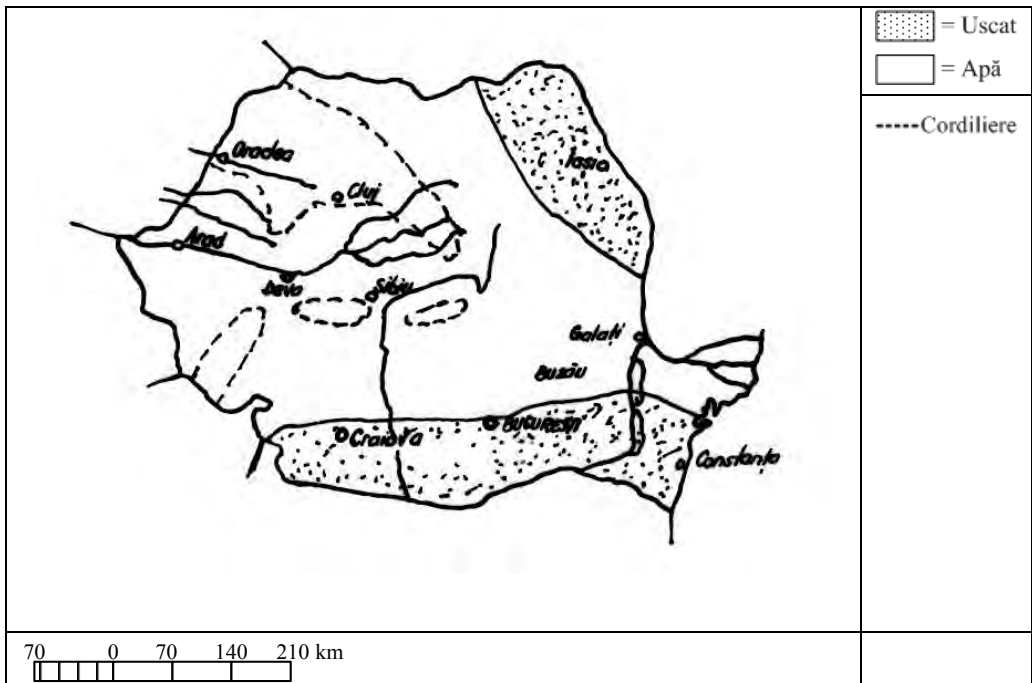
Foto 2. Situația în Paleozoicul inferior
