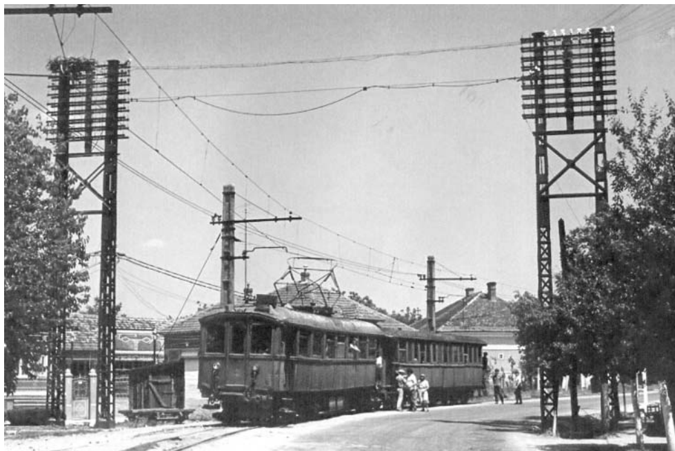
Motorul electric în stația Covăsânț-centru
