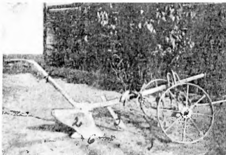
1. Coarnele 2. Cormanul 3. Cioroslea 4. Grindeiul 5. Rocitele 6. Feru plugului 7. Scărița (sub grindei, cu care se regulează adâncimea brazdei)
